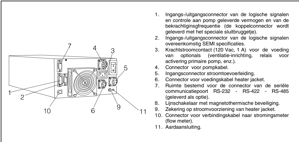
Achterpaneel van de controllers 969-9448 en 969-9449
